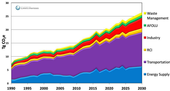
图 1 墨西哥下加利福尼亚州未来照常情景排放增长情况
